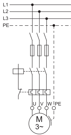
DOL
